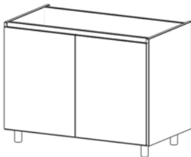
Module met 2 draaideuren + 1 binnenplank 1206mm
