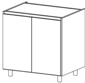
Module met 2 draaideuren + 1 binnenplank 912mm
